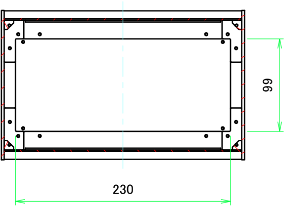
B-B ( 1 : 4 )
