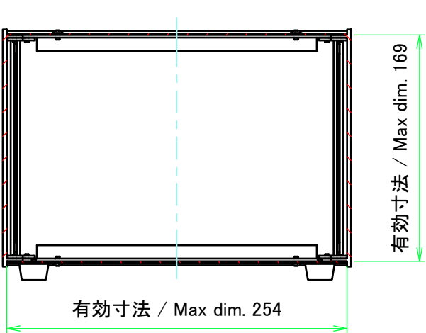
C-C ( 1 : 4 )
