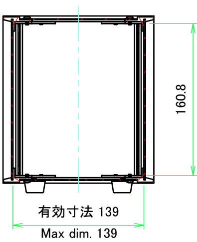
A-A ( 1 : 4 )
