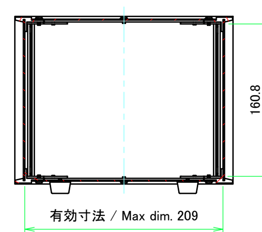
A-A ( 1 : 4 )
