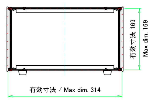
C-C ( 1 : 5 )
