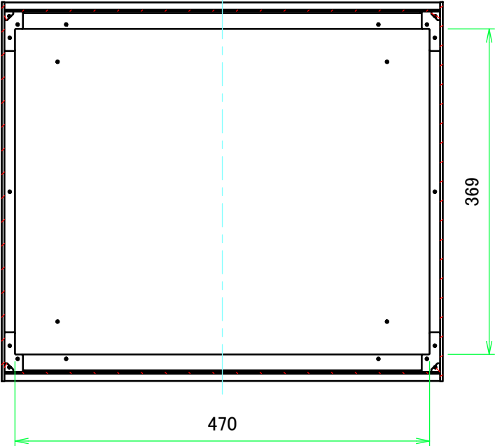
B-B ( 1 : 6 )
