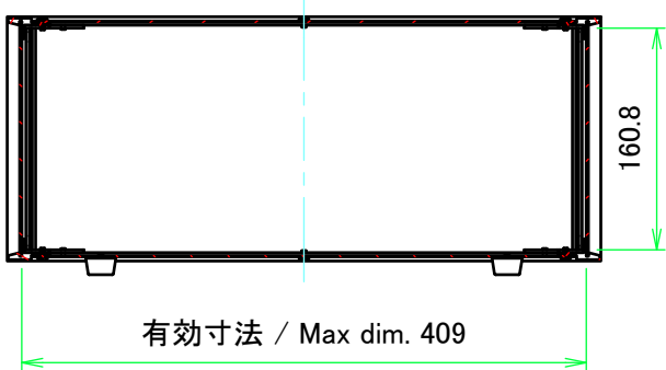
A-A ( 1 : 6 )
