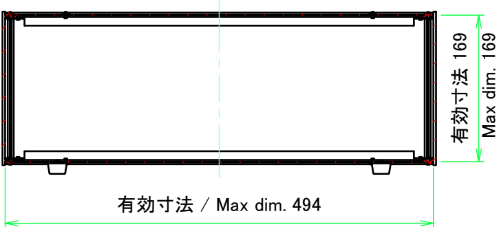
C-C ( 1 : 6 )
