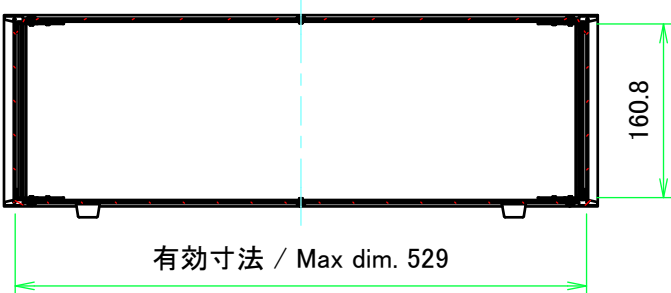
A-A ( 1 : 7 )
