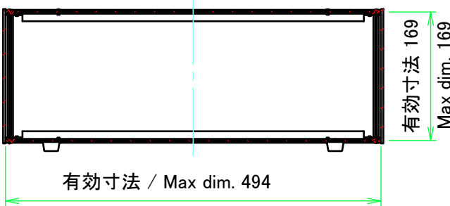
C-C ( 1 : 7 )
