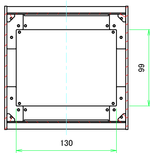
B-B ( 1 : 3 )
