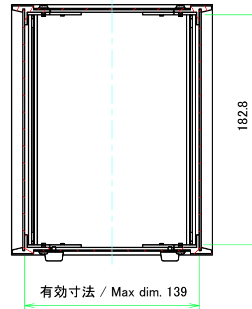
A-A ( 1 : 3 )
