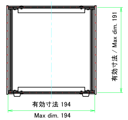
C-C ( 1 : 4 )
