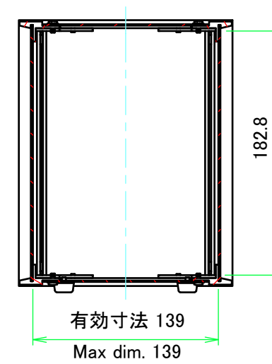
A-A ( 1 : 4 )
