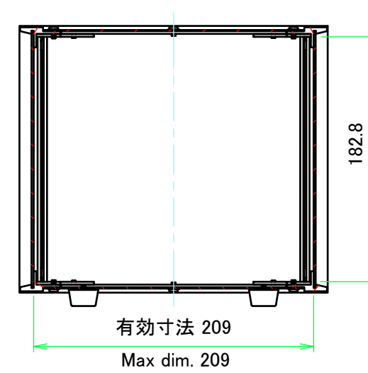
A-A ( 1 : 4 )
