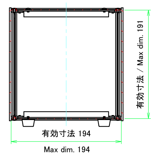
C-C ( 1 : 4 )
