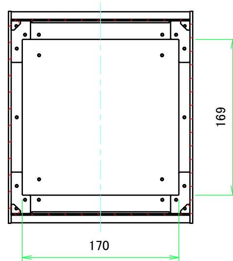
B-B ( 1 : 4 )
