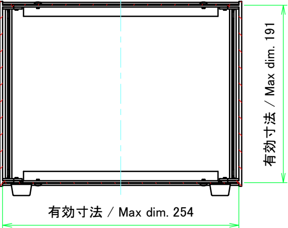
C-C ( 1 : 4 )
