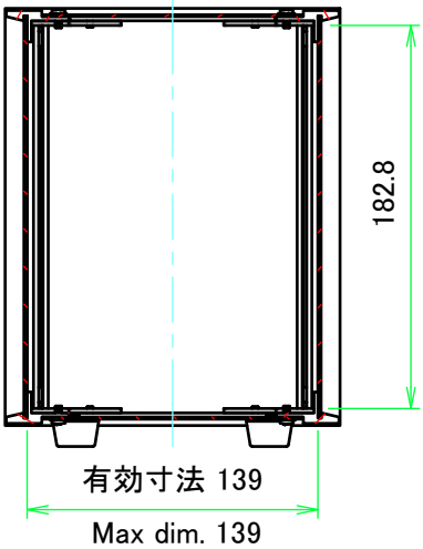
A-A ( 1 : 4 )
