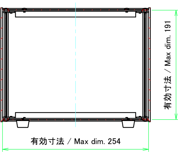
C-C ( 1 : 4 )
