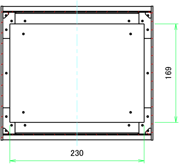
B-B ( 1 : 4 )
