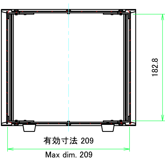
A-A ( 1 : 4 )
