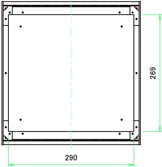
B-B ( 1 : 5 )
