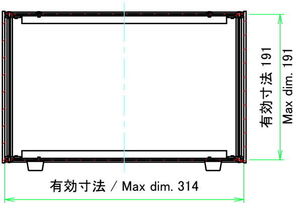
C-C ( 1 : 5 )
