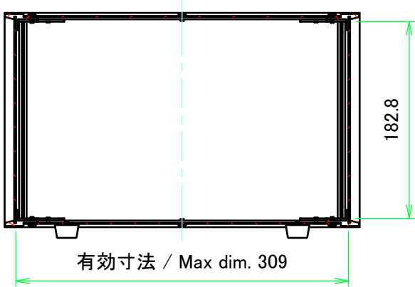
A-A ( 1 : 5 )
