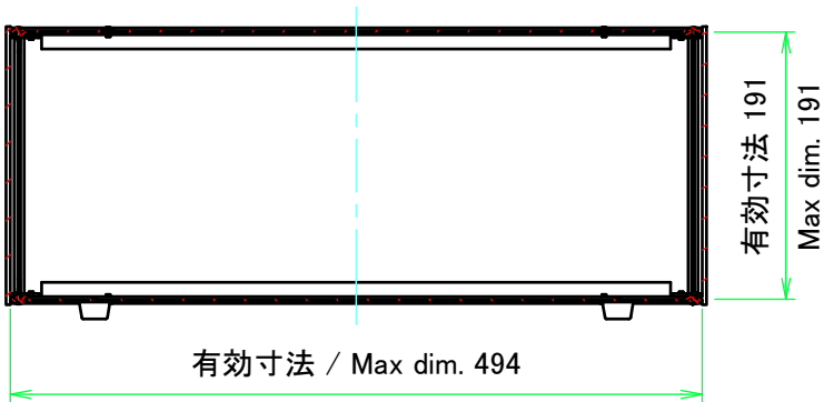
C-C ( 1 : 6 )
