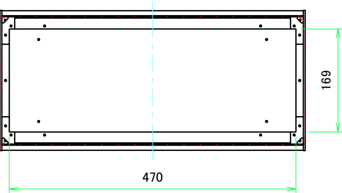
B-B ( 1 : 6 )
