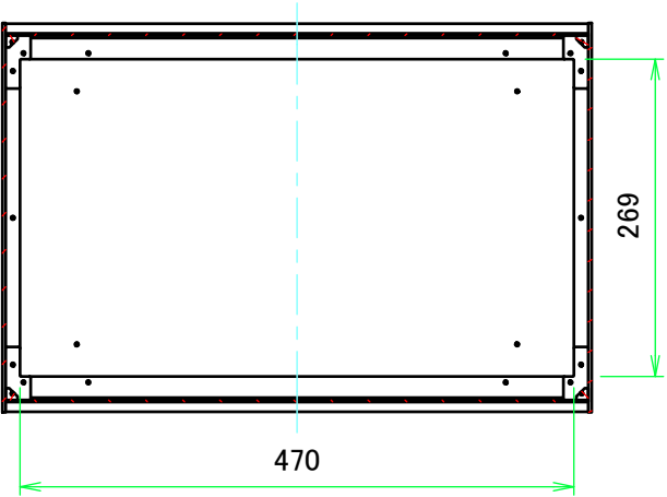
B-B ( 1 : 7 )
