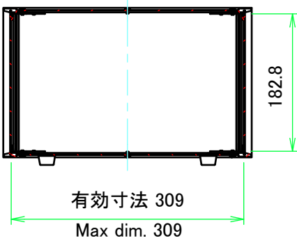
A-A ( 1 : 7 )
