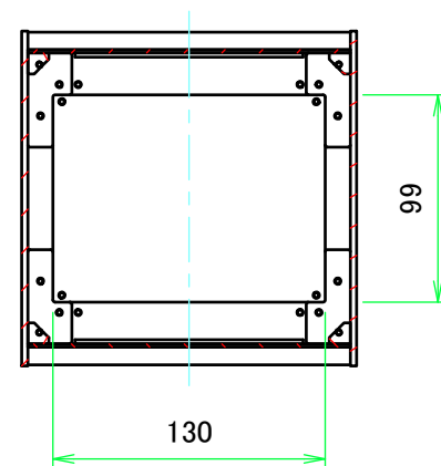
B-B ( 1 : 4 )
