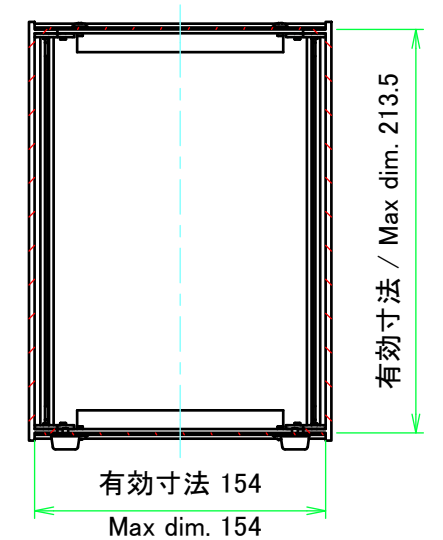
C-C ( 1 : 4 )
