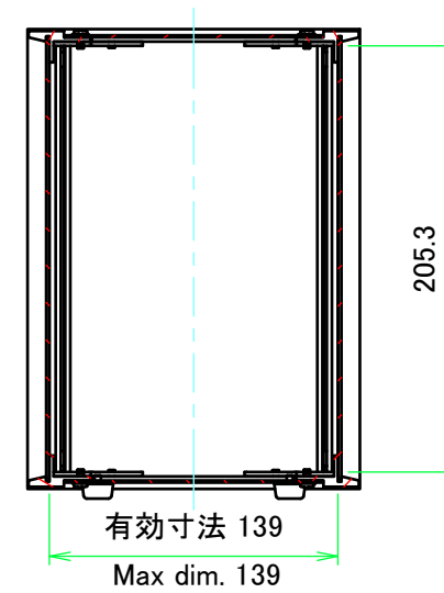
A-A ( 1 : 4 )
