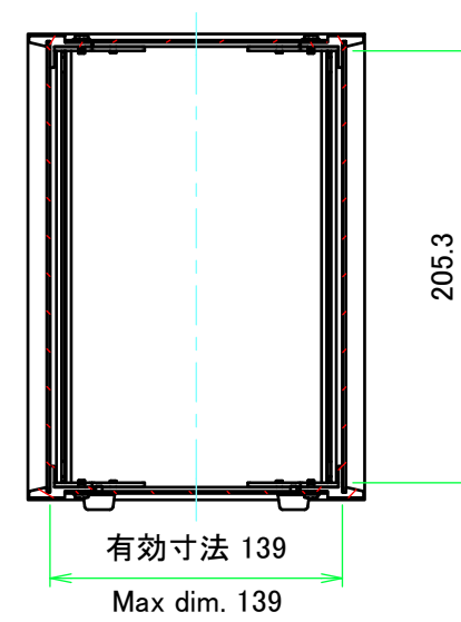
A-A ( 1 : 4 )
