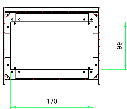
B-B ( 1 : 4 )
