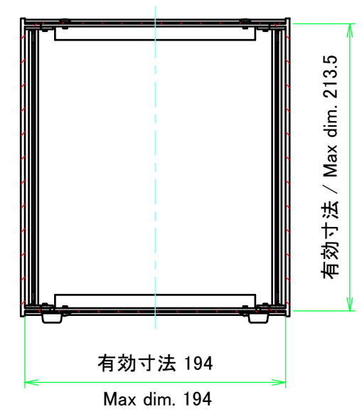
C-C ( 1 : 4 )
