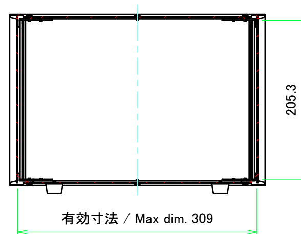
A-A ( 1 : 5 )
