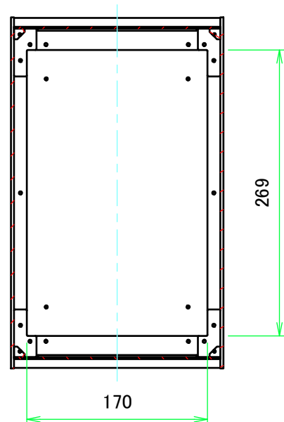
B-B ( 1 : 5 )
