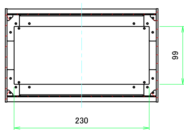
B-B ( 1 : 4 )
