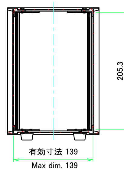
A-A ( 1 : 4 )
