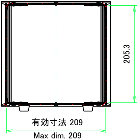
A-A ( 1 : 5 )
