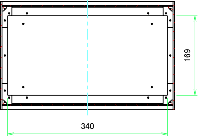
B-B ( 1 : 5 )
