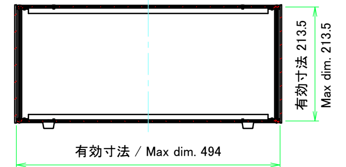
C-C ( 1 : 7 )
