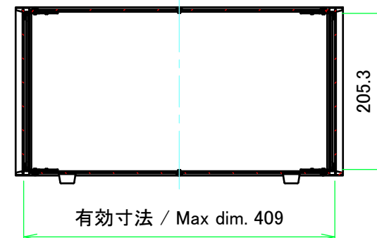
A-A ( 1 : 7 )
