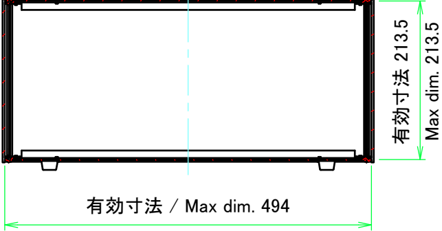
C-C ( 1 : 7 )
