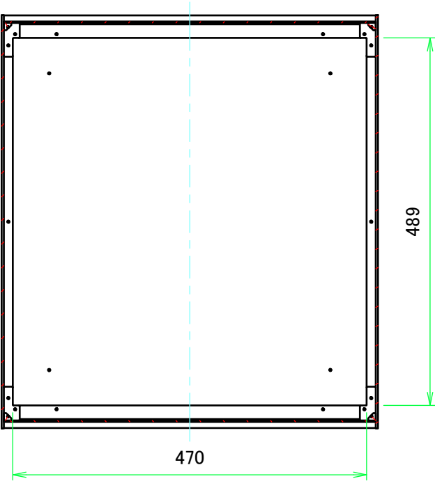
B-B ( 1 : 7 )
