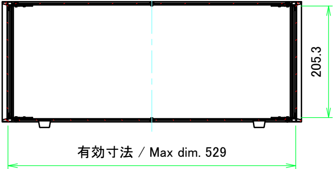
A-A ( 1 : 7 )
