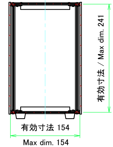
C-C ( 1 : 5 )
