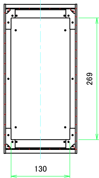
B-B ( 1 : 5 )
