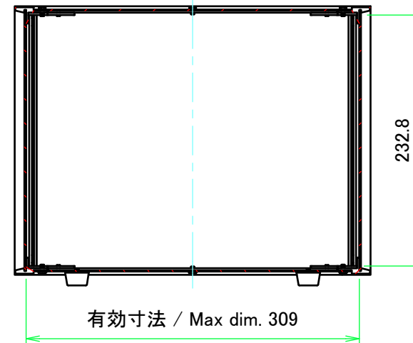
A-A ( 1 : 5 )
