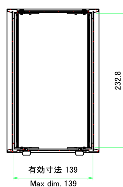
A-A (1:4)
