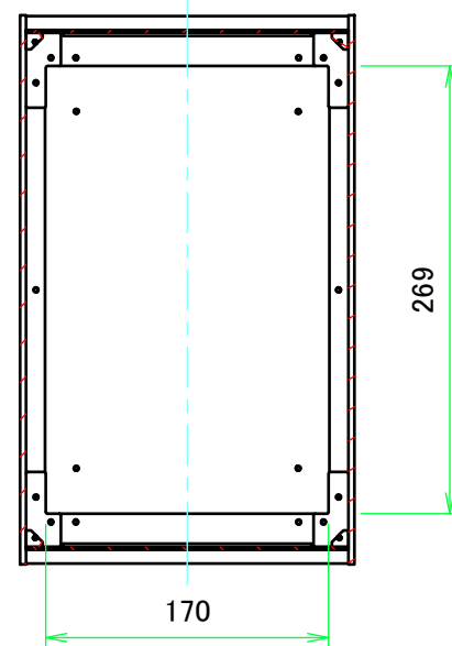
B-B ( 1 : 5 )
