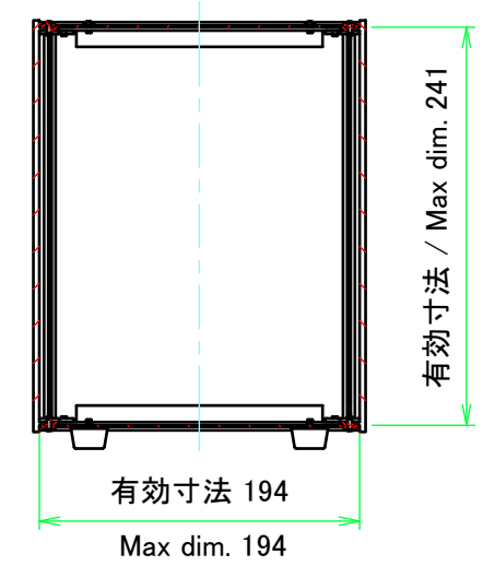
C-C ( 1 : 5 )
