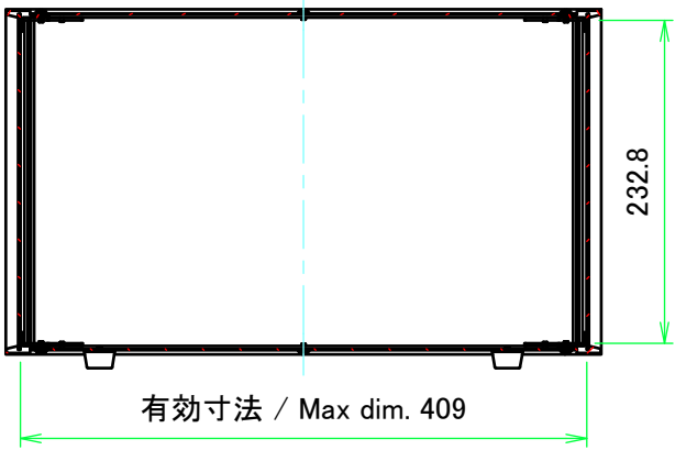
A-A ( 1 : 6 )
