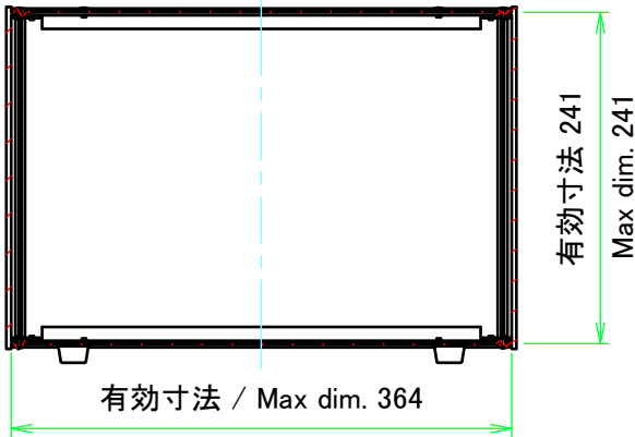
C-C ( 1 : 6 )
