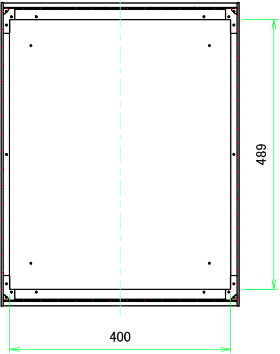
B-B ( 1 : 7 )
