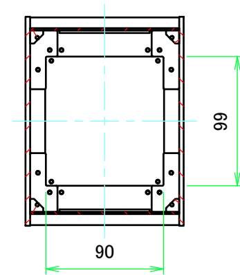
B-B ( 1 : 4 )
