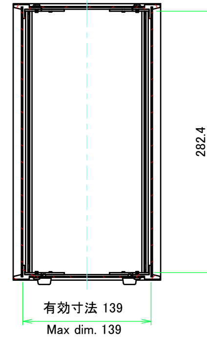
A-A ( 1 : 4 )
