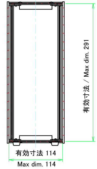
C-C ( 1 : 4 )
