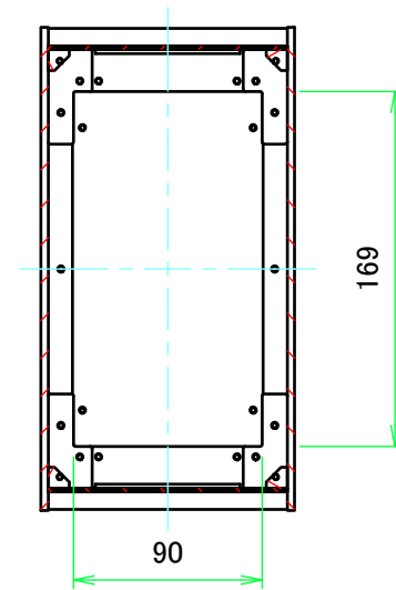
B-B ( 1 : 4 )
