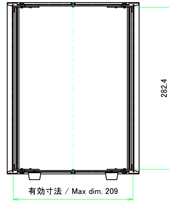
A-A ( 1 : 4 )
