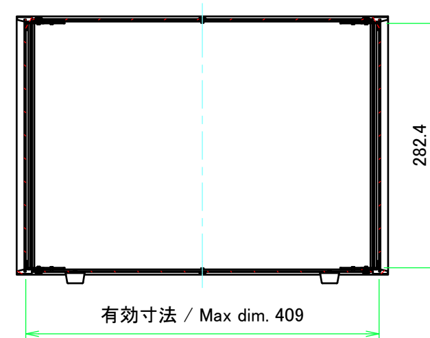
A-A (1:6)
