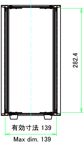
A-A ( 1 : 5 )
