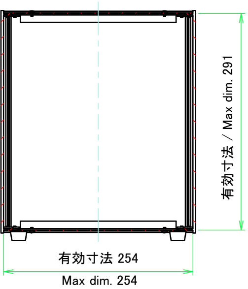
C-C ( 1 : 5 )
