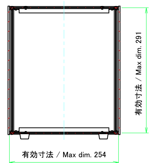
C-C ( 1 : 5 )
