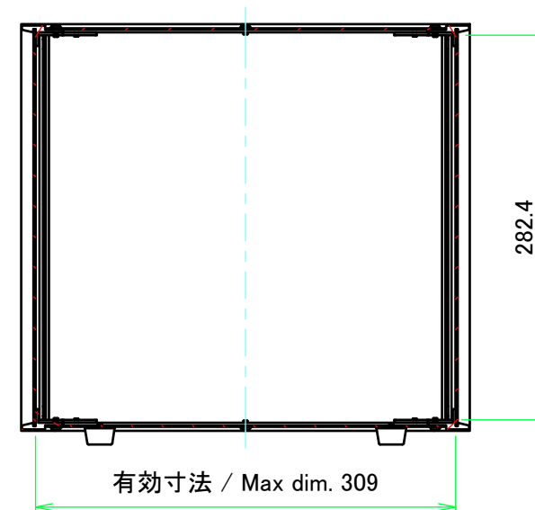
A-A ( 1 : 5 )
