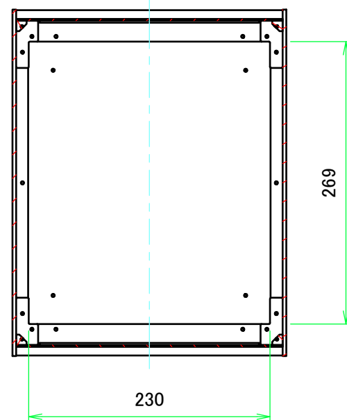
B-B ( 1 : 5 )
