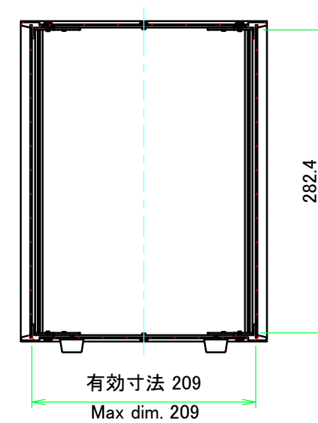
A-A (1:5)
