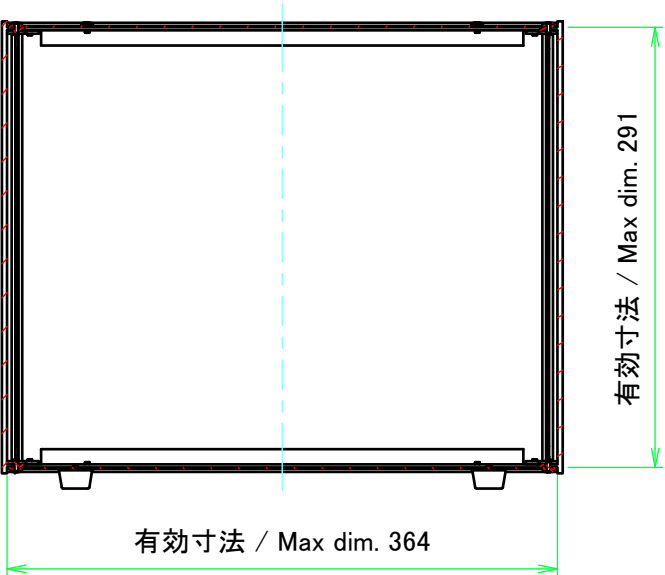
C-C ( 1 : 5 )
