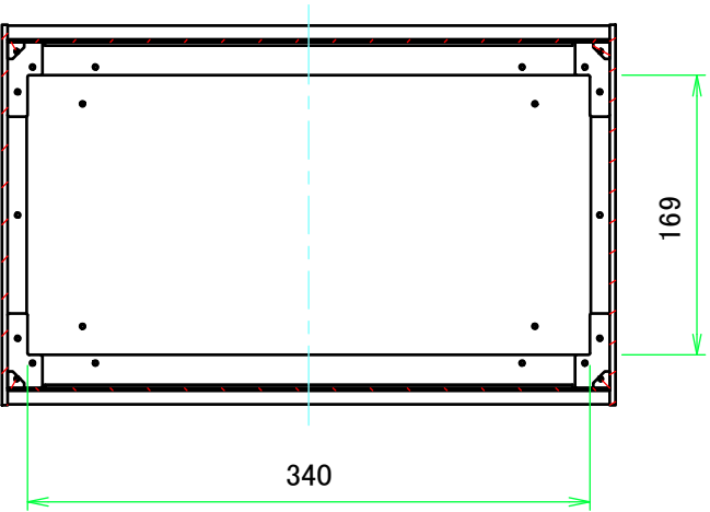
B-B ( 1 : 5 )
