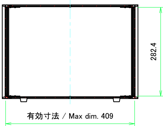
A-A ( 1 : 7 )
