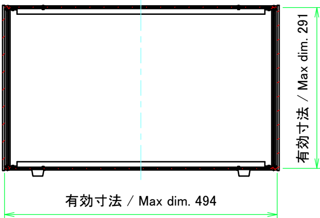
C-C ( 1 : 7 )
