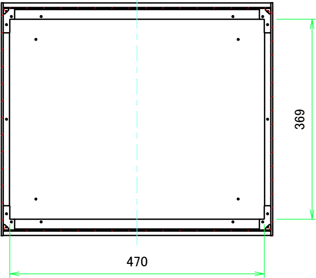
B-B ( 1 : 7 )
