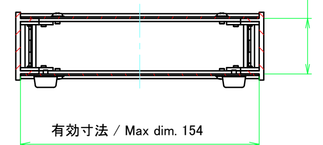
C-C ( 1 : 2.5 )
