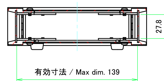
A-A ( 1 : 2.5 )
