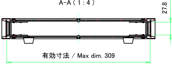
A-A ( 1 : 4 )
