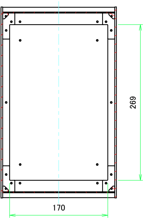
B-B ( 1 : 4 )
