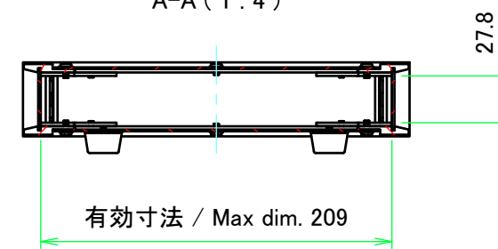
A-A ( 1 : 4 )
