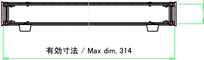
C-C ( 1 : 4 )
