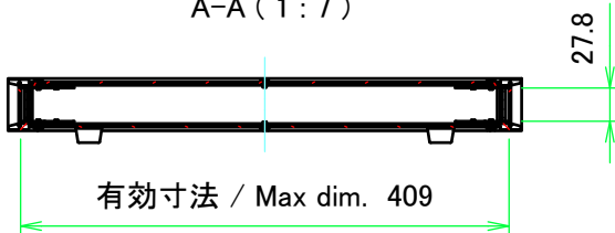
A-A ( 1 : 7 )
