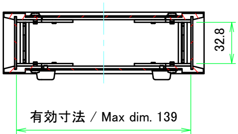
A-A (1:3)
