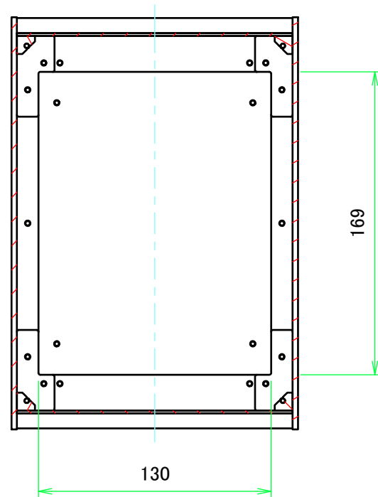
B-B ( 1 : 3 )
