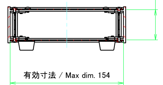
C-C ( 1 : 3 )
