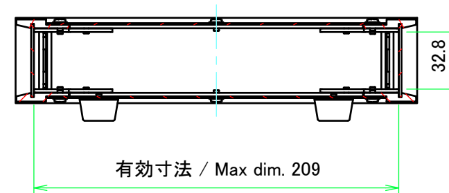
A-A ( 1 : 3 )
