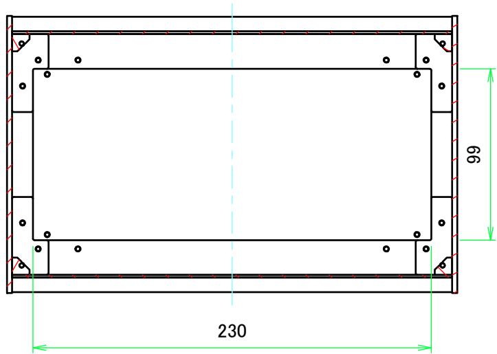
B-B ( 1 : 3 )
