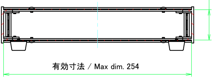
C-C ( 1 : 3 )
