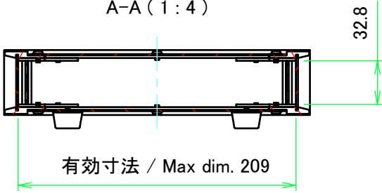
A-A (1:4)
