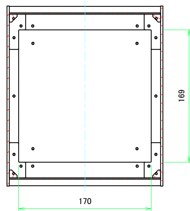
B-B ( 1 : 3 )
