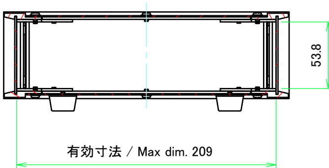
A-A ( 1 : 3 )
