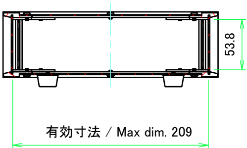
A-A ( 1 : 4 )
