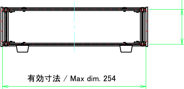
C-C ( 1 : 4 )
