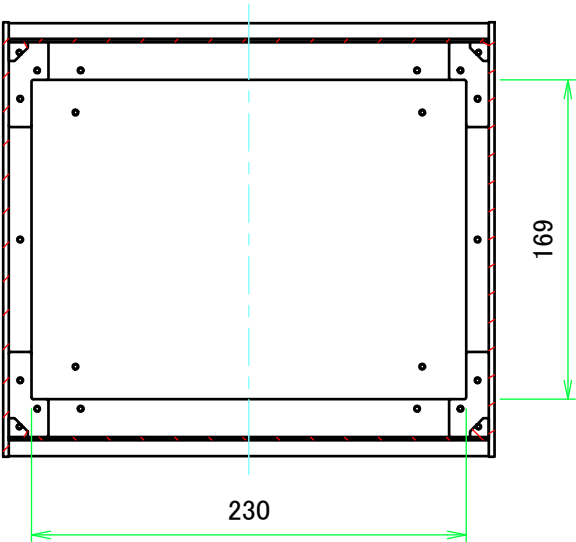
B-B ( 1 : 4 )
