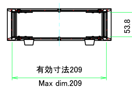
A-A ( 1 : 5 )
