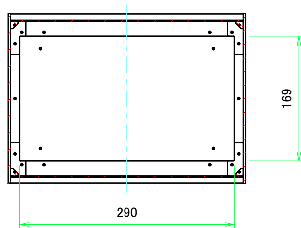
B-B ( 1 : 5 )
