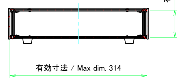
C-C ( 1 : 5 )
