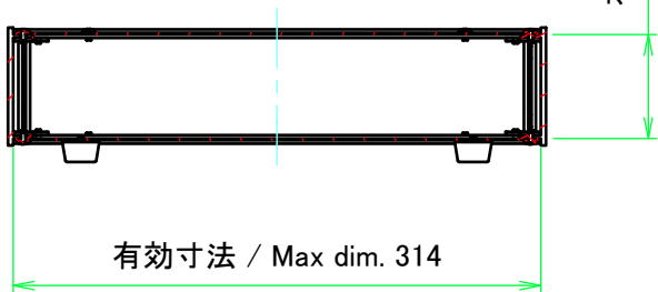
C-C ( 1 : 5 )
