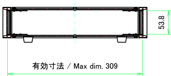
A-A ( 1 : 5 )
