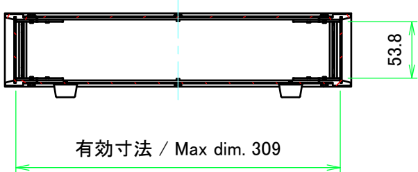
A-A ( 1 : 5 )
