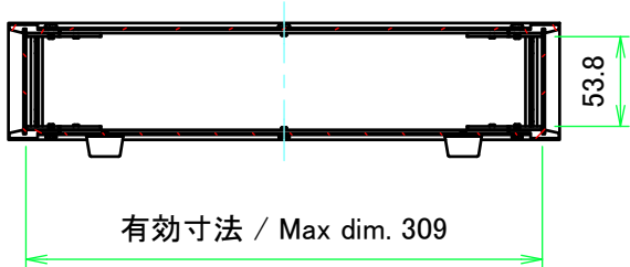
A-A ( 1 : 5 )
