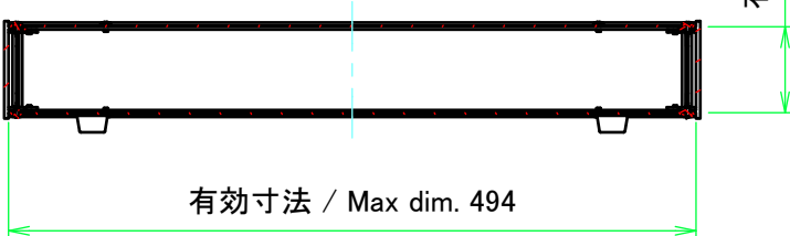
C-C ( 1 : 6 )
