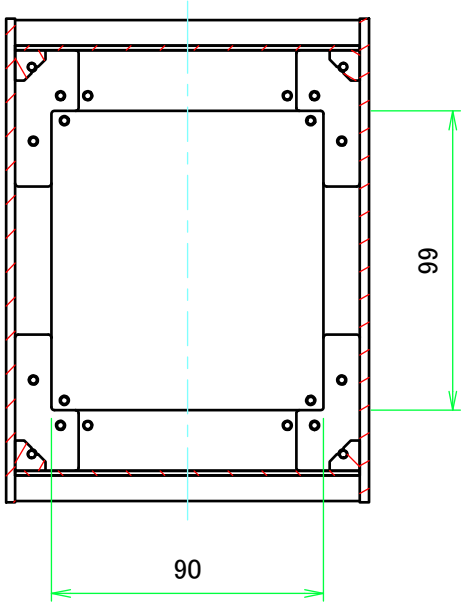
B-B ( 1 : 2.5 )
